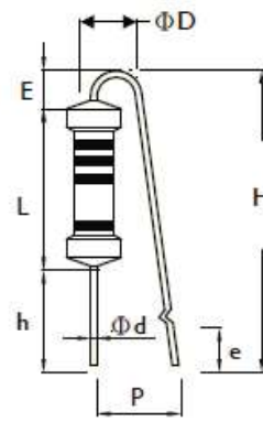
FFK TYPE
